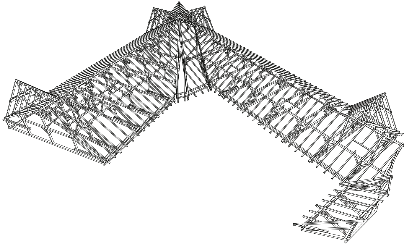
PŮVODNÍ STAV
